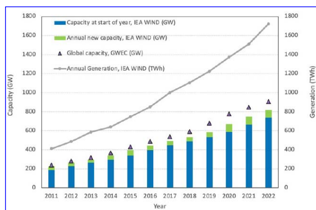
図2 2011～2022暦年の風力発電の導入トレンド
